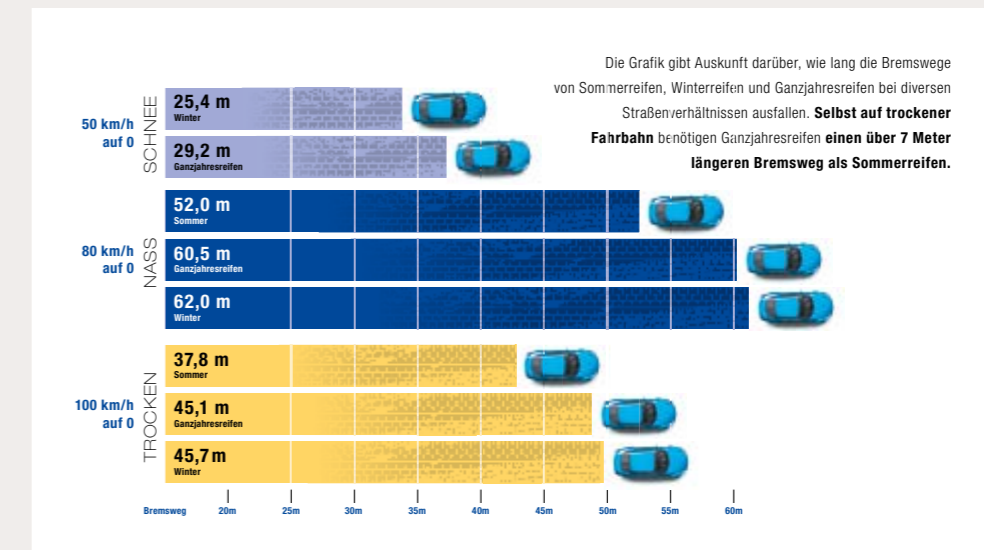
Quelle: ACE-Reifentest 09/2016
